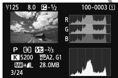
直方圖
